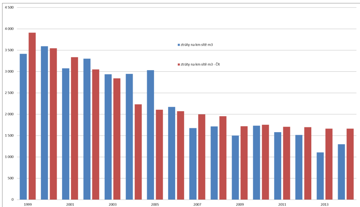
Graf č. 8 – Přehled vývoje ztrát vody na km sítě v tis. m3 – VAK Náchod, a.s.
