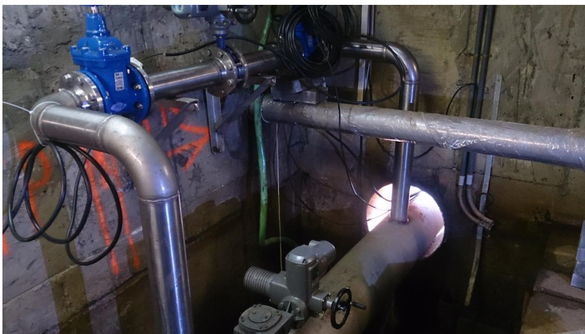
Obrázek č. 3 – Pohled na armaturní komoru – Broumovský uzel, Teplice nad Metují
