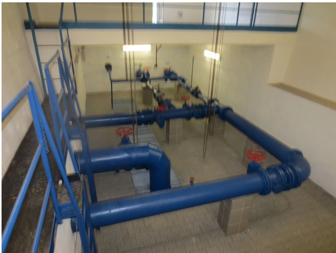
obrázek č.7 Pohled na armaturní komoru VDJ Vysokov
